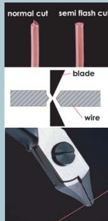
Precision Pliers
